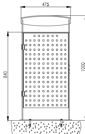
Frontansicht Ausführung zum Aufschauben
