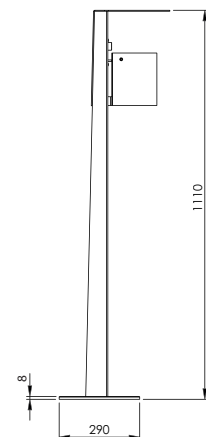
7070 S-00 Seitenansicht
