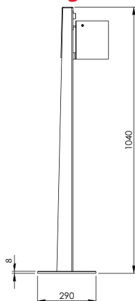
7067 S-00 Seitenansicht
