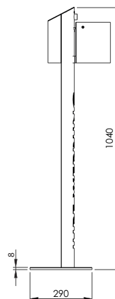
7067 S-01 Seitenansicht
