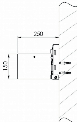
Wandbefestigung
