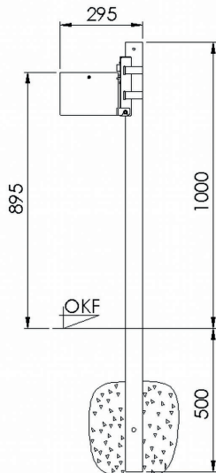
Pfostenbefestigung
