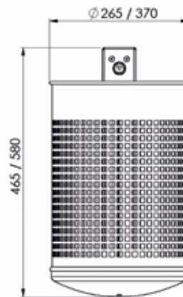
Frontansicht
