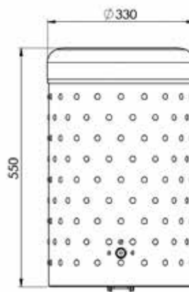
Frontansicht
