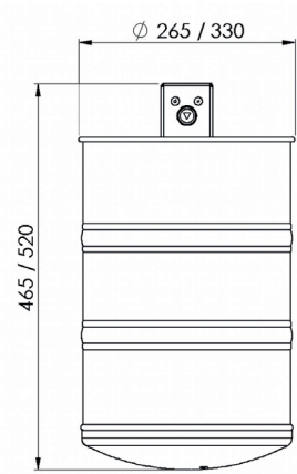
Frontansicht
