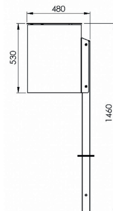
Seitenansicht
